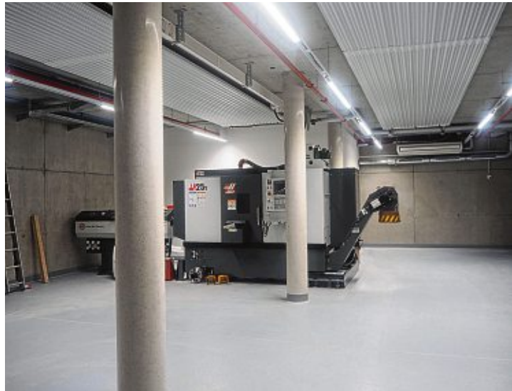
Die neue CNC-Drehmaschine wartet bereits auf ihren Einsatz. Die weiteren Produktionsgeräte werden in den kommenden Wochen umgezogen.
